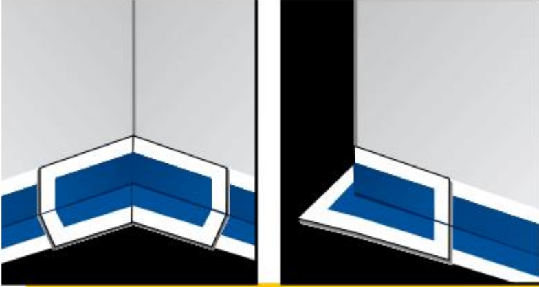
İç köşe profillerin yerleştirilmesi
